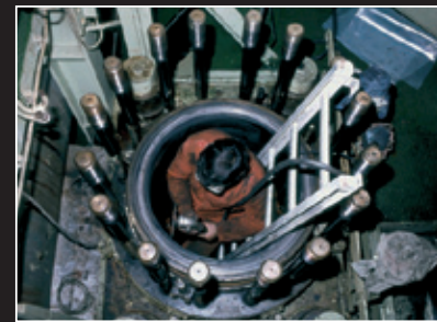
Nahře: Broušení vložky hlavního motoru, m/s Slapy, 27. 7. 1982, Říječna
